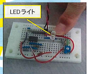
心拍センサー(工作品)
